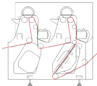
iFlex per etichette UV/UV Led – Aria calda
